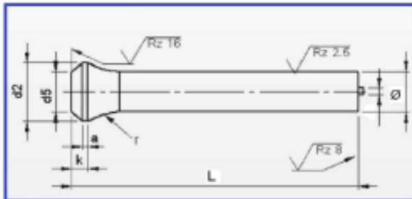
Forma de pedido: 831E-Ø10x80
