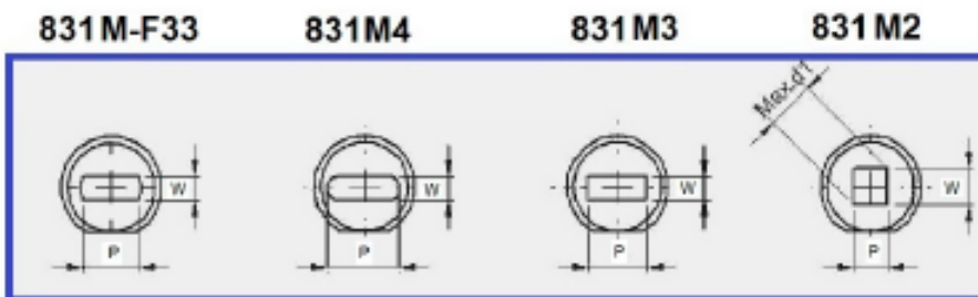
Forma de pedido: 831M4-Ø10 P=8 W=3.1 L=100
